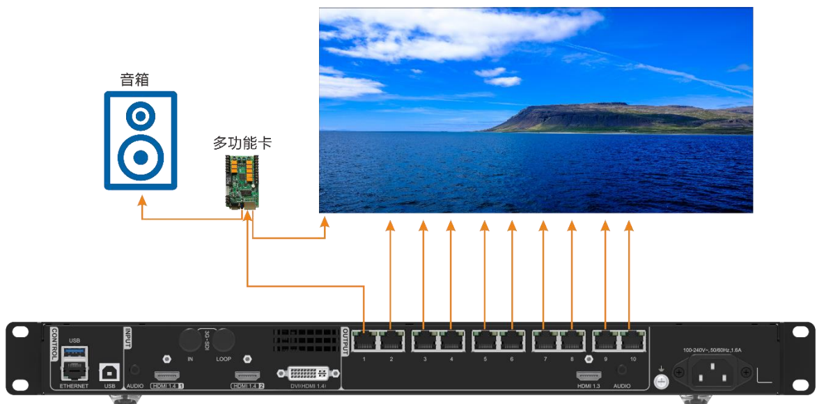
图5-39 音频输出连接（多功能卡连接）
