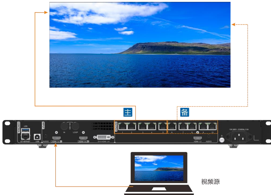
图5-22 网口备份连线图
