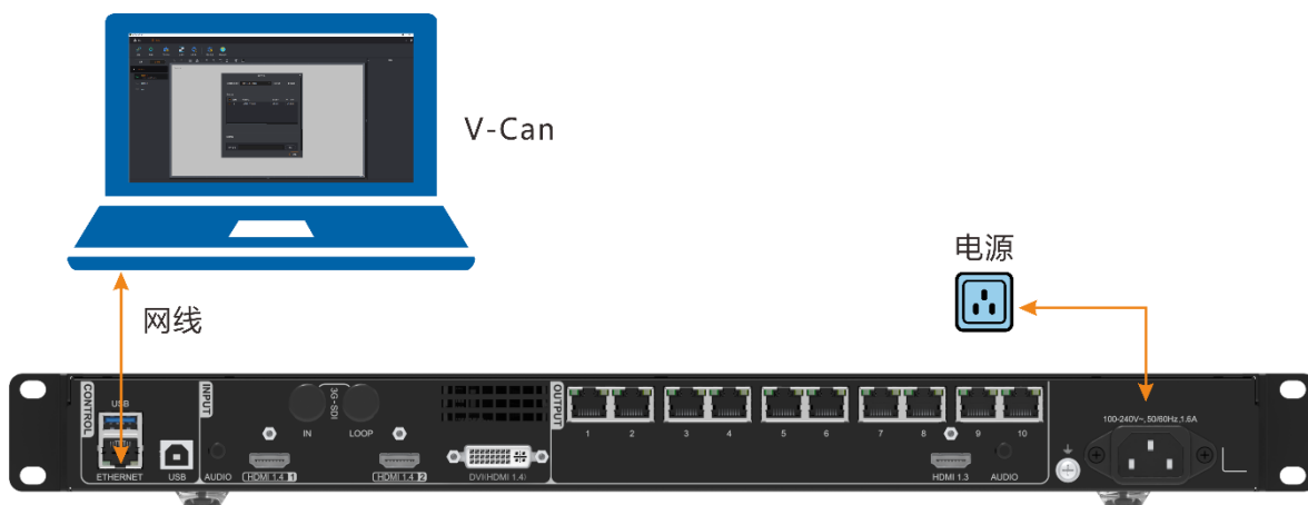
图6-1 固件升级硬件连接
