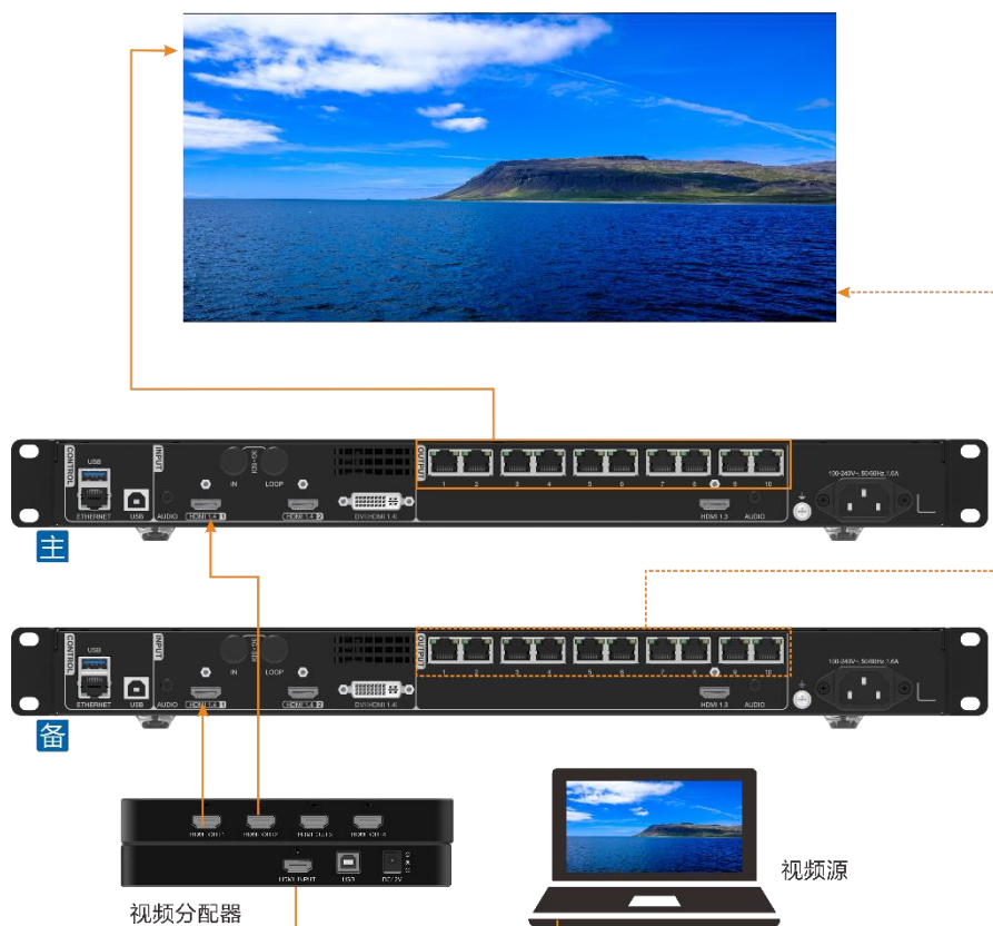
图5-20 设备热备份连接图
